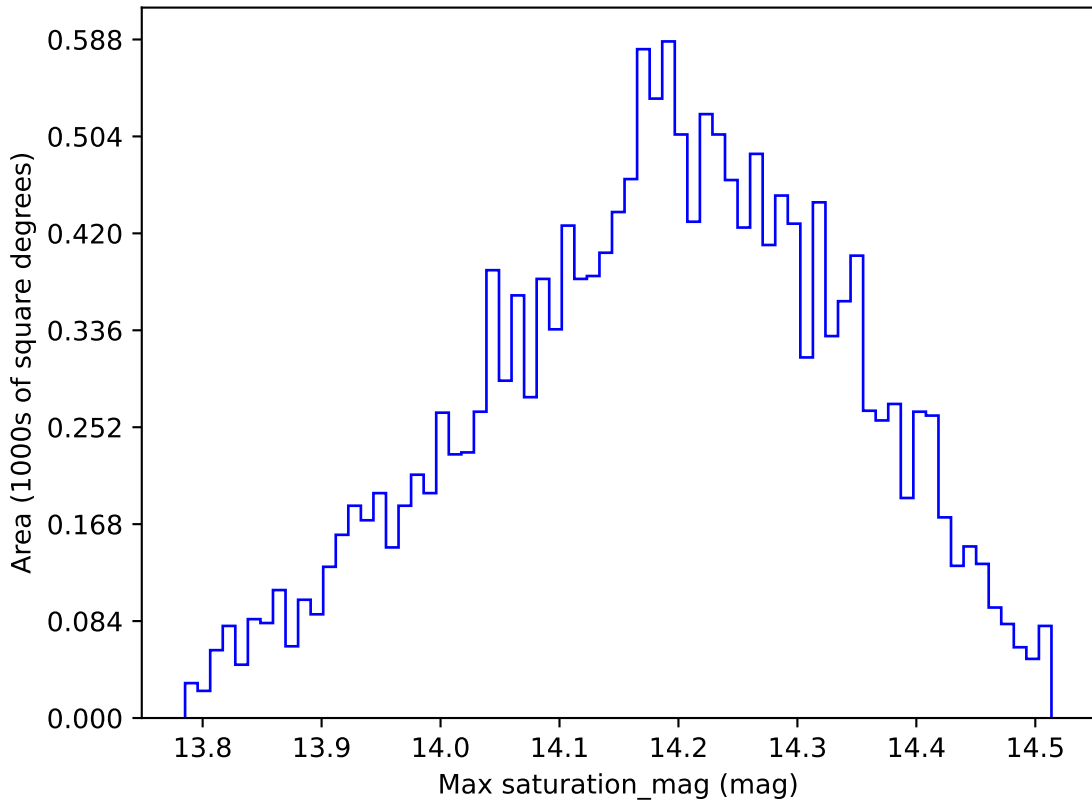
noroll_v3.4_10yrs WFD y band: Max saturation_mag
