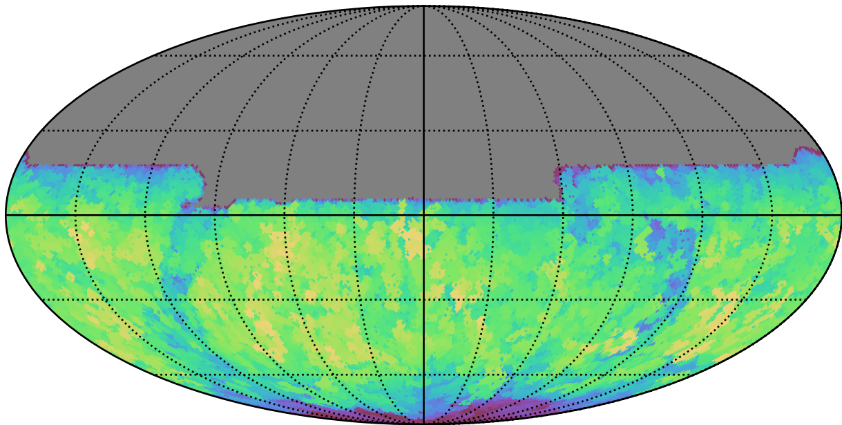
noroll_v3.4_10yrs All sky y band: Max saturation_mag
