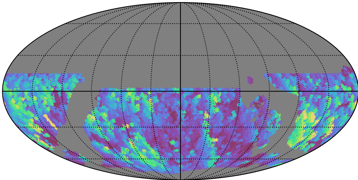
noroll_v3.4_10yrs WFD y band: Max normairmass
