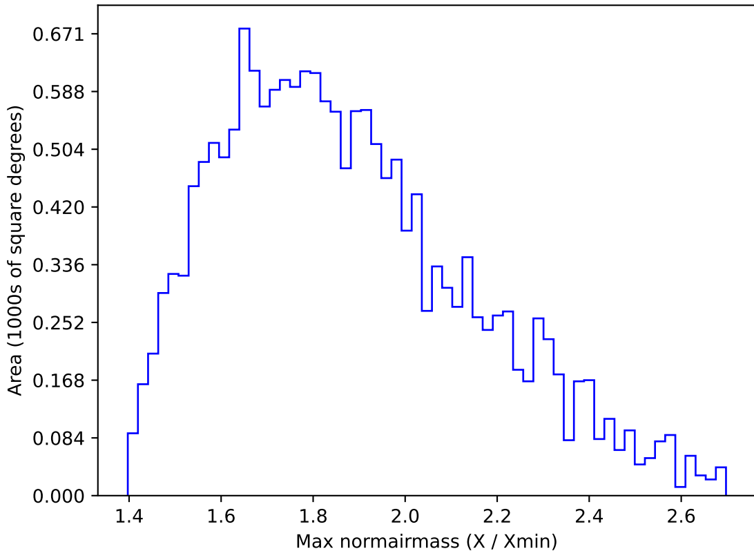
noroll_v3.4_10yrs WFD y band: Max normairmass
