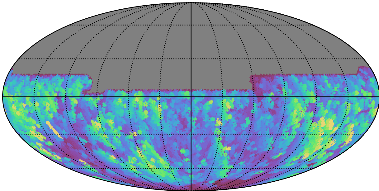
noroll_v3.4_10yrs All sky y band: Max normairmass
