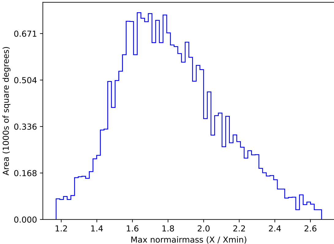
noroll_v3.4_10yrs All sky y band: Max normairmass
