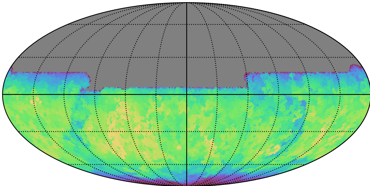
noroll_v3.4_10yrs All sky y band: Max fiveSigmaDepth
