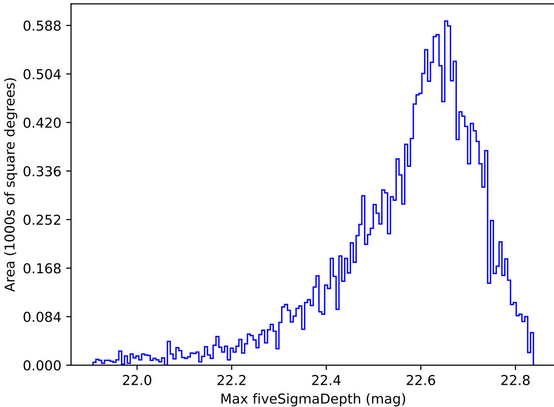
noroll_v3.4_10yrs All sky y band: Max fiveSigmaDepth
