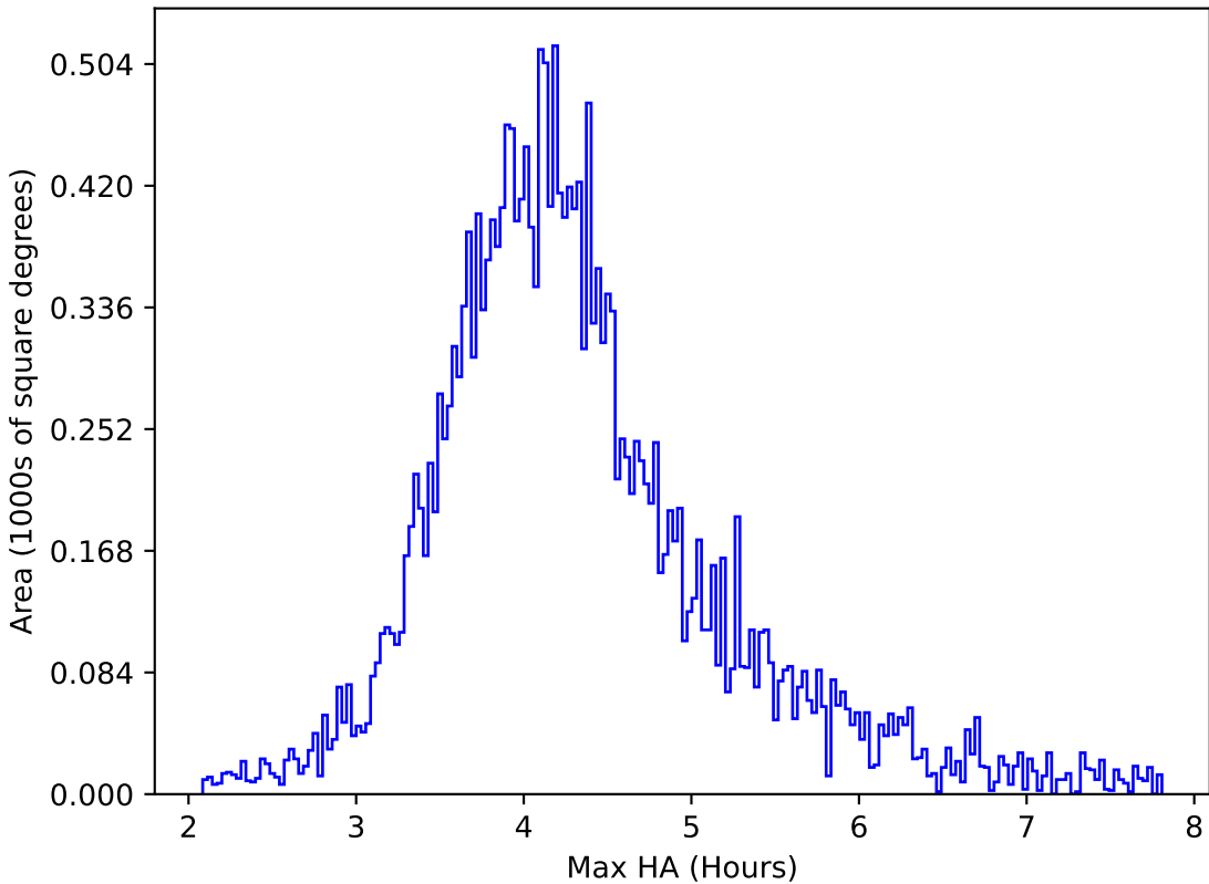
noroll_v3.4_10yrs All sky y band: Max HA
