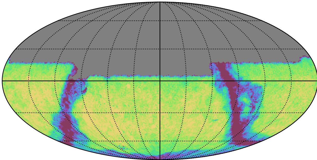
noroll_v3.4_10yrs Yr 1 y band: Exgal_CoaddM5
