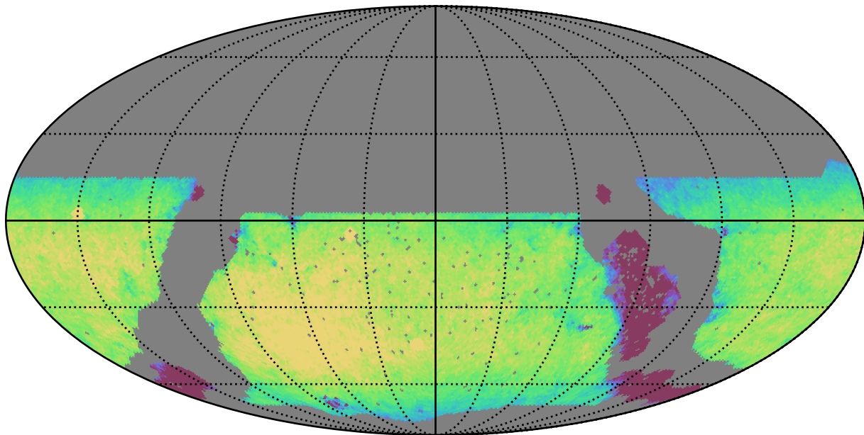
noroll_v3.4_10yrs WFD y band: Exgal_CoaddM5
