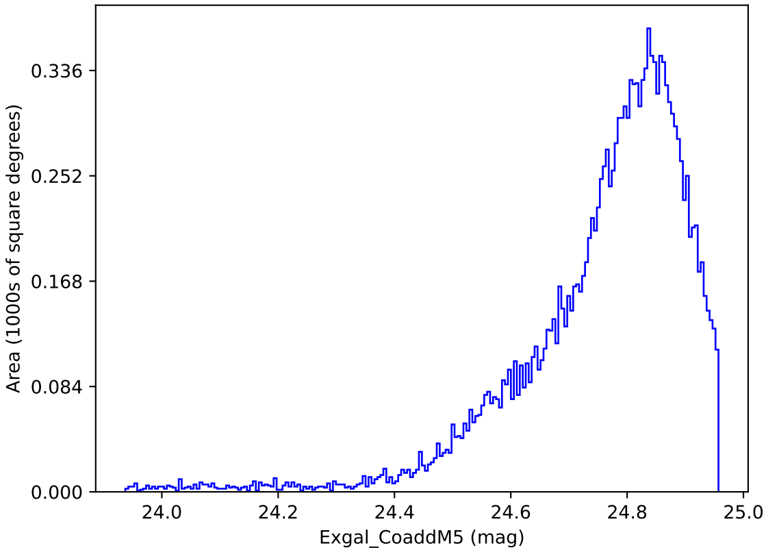
noroll_v3.4_10yrs WFD y band: Exgal_CoaddM5
