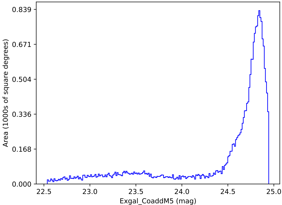
noroll_v3.4_10yrs All sky y band: Exgal_CoaddM5
