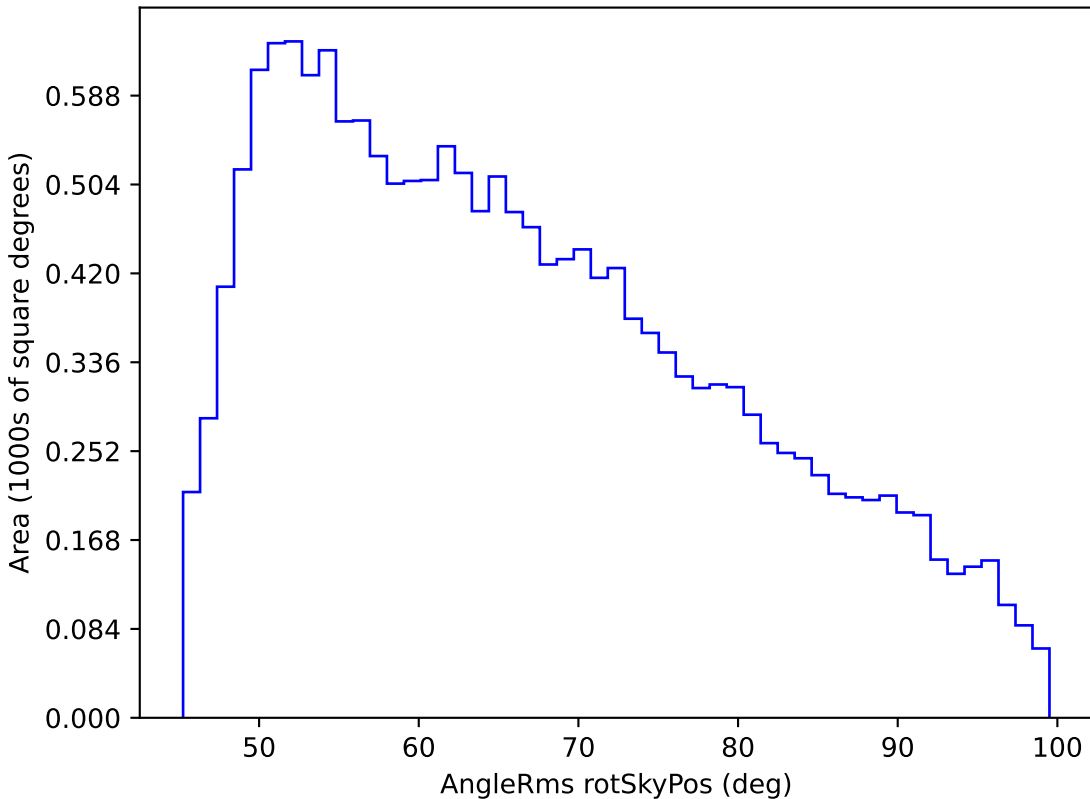
noroll_v3.4_10yrs WFD y band: AngleRms rotSkyPos
