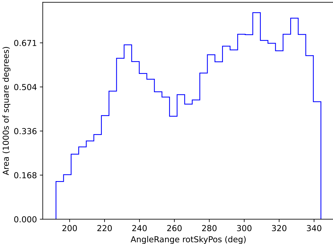
noroll_v3.4_10yrs WFD z band: AngleRange rotSkyPos
