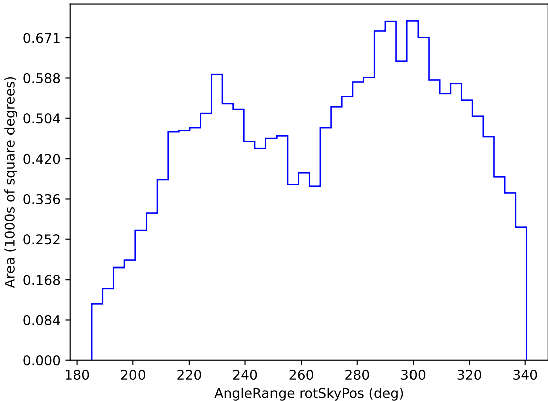
noroll_v3.4_10yrs WFD y band: AngleRange rotSkyPos
