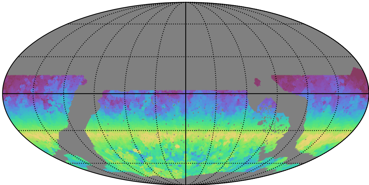
noroll_v3.4_10yrs WFD r band: AngleRange rotSkyPos
