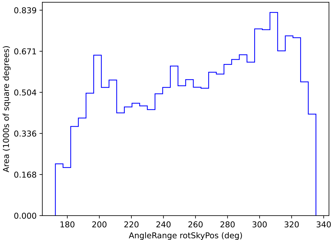
noroll_v3.4_10yrs WFD g band: AngleRange rotSkyPos
