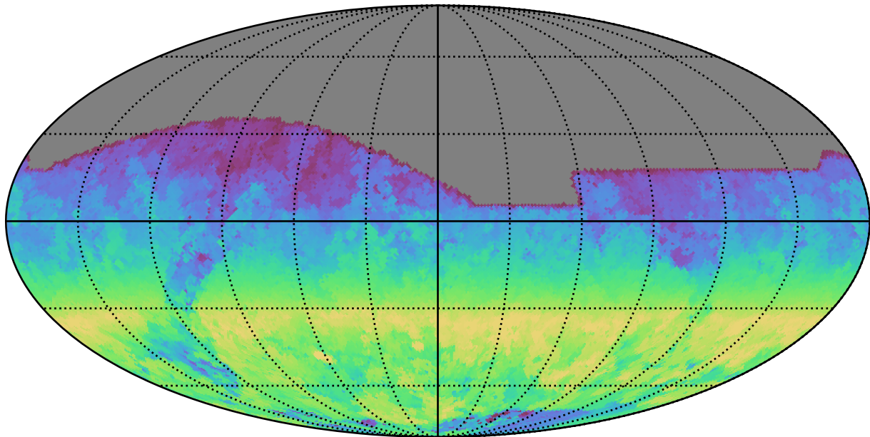
noroll_v3.4_10yrs All sky z band: AngleRange rotSkyPos
