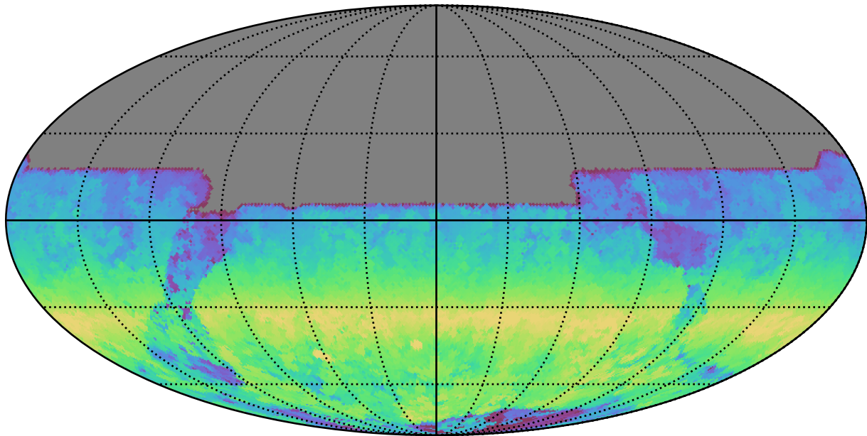
noroll_v3.4_10yrs All sky y band: AngleRange rotSkyPos
