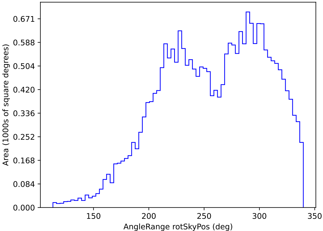
noroll_v3.4_10yrs All sky y band: AngleRange rotSkyPos
