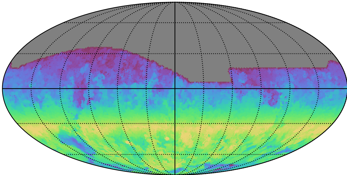
noroll_v3.4_10yrs All sky i band: AngleRange rotSkyPos
