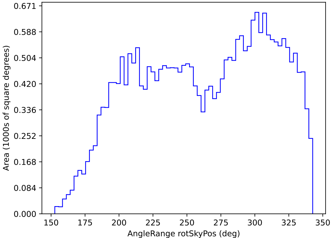
noroll_v3.4_10yrs All sky i band: AngleRange rotSkyPos
