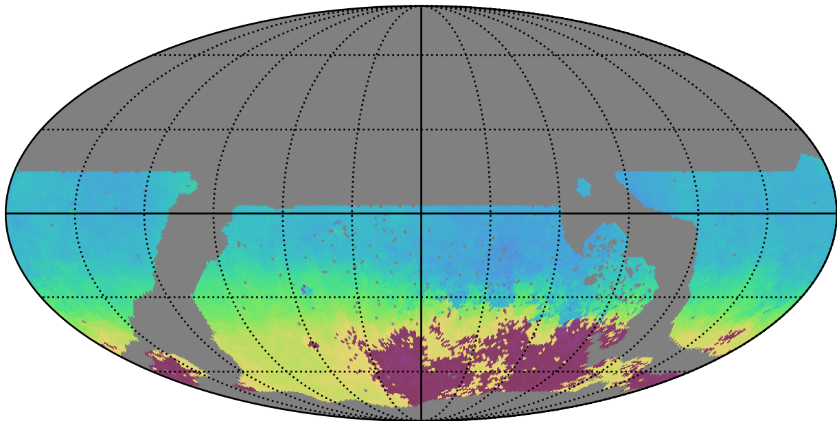
noroll_v3.4_10yrs WFD y band: AngleMean rotSkyPos
