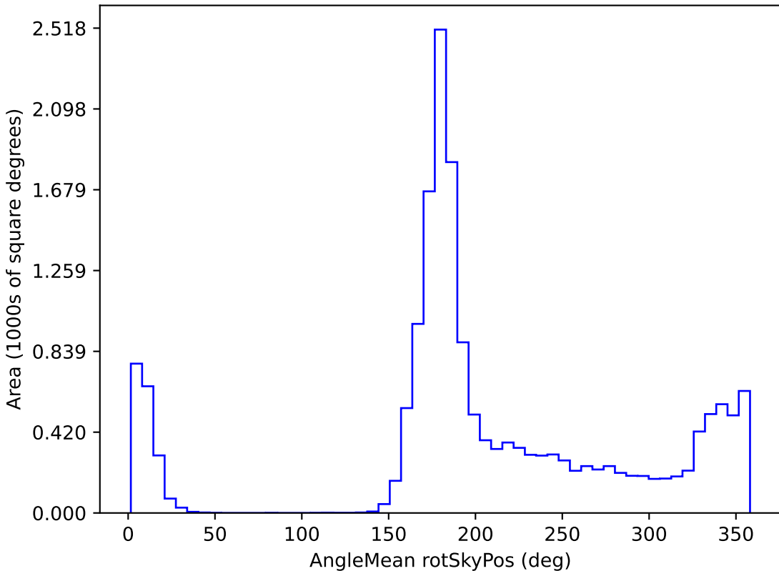
noroll_v3.4_10yrs WFD y band: AngleMean rotSkyPos
