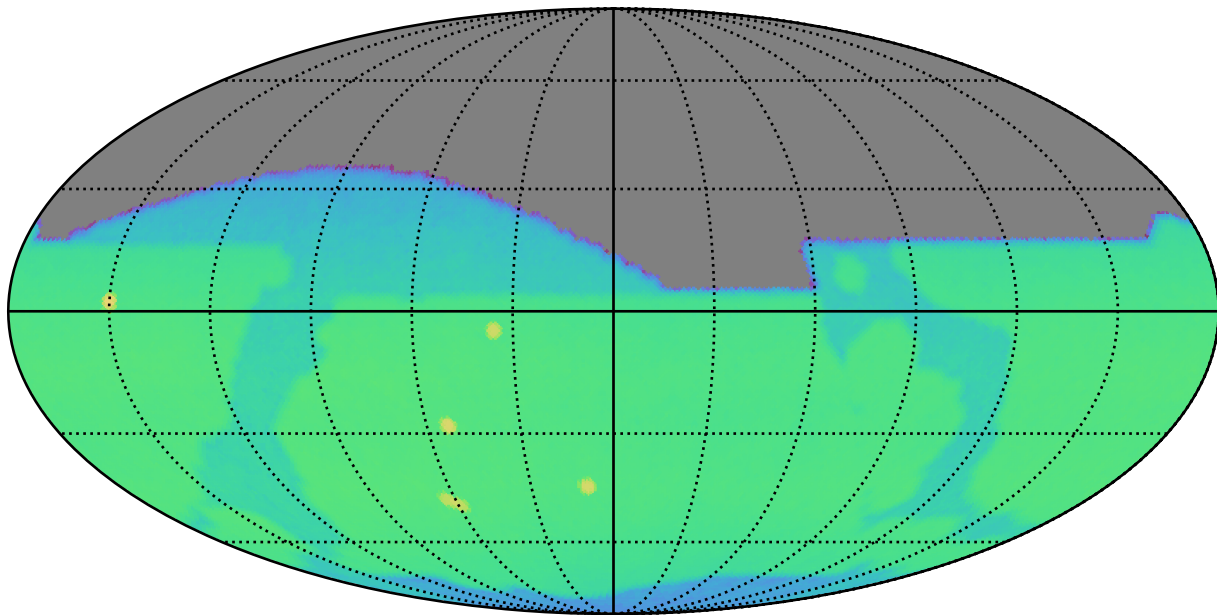
noroll_v3.4_10yrs i: CoaddM5
