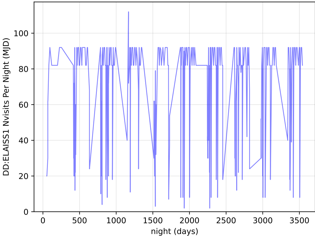
noroll_v3.4_10yrs all bands: DD:ELAISS1 Nvisits Per Night
