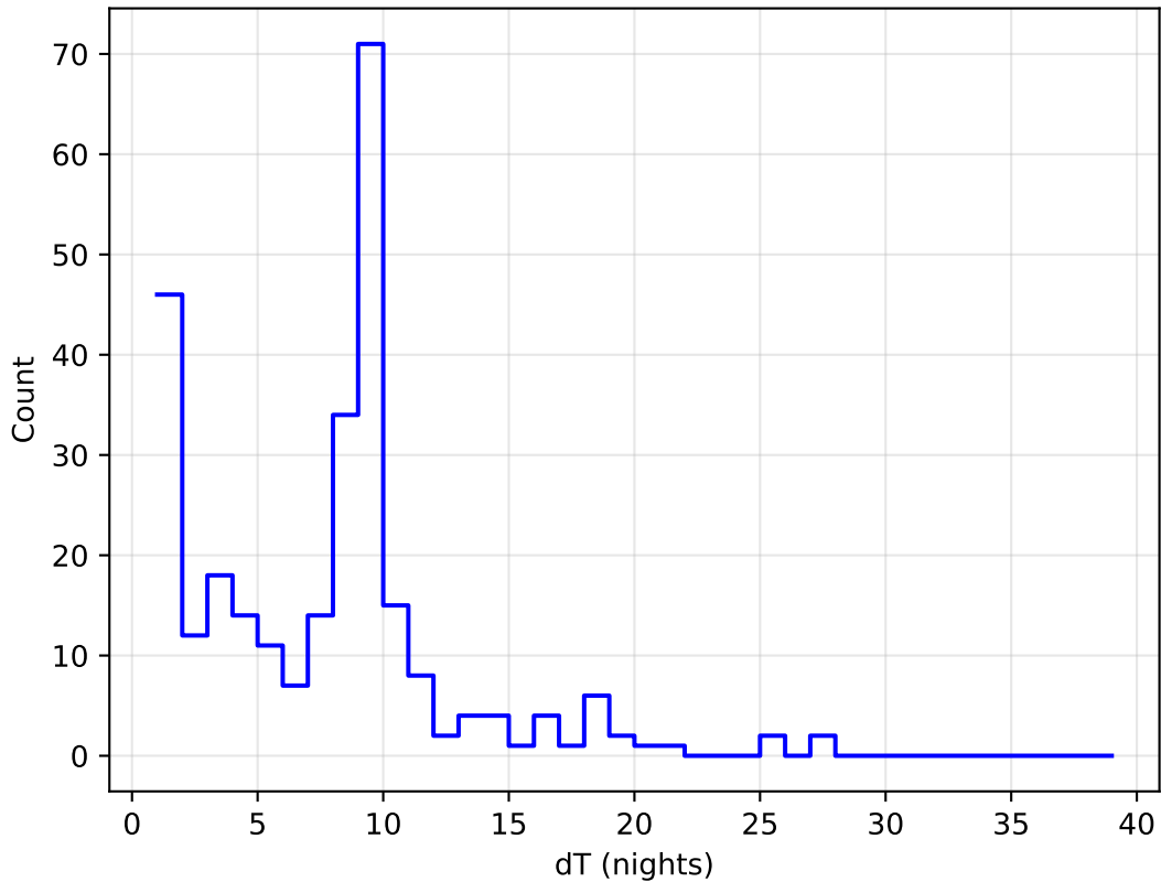
noroll_v3.4_10yrs all bands: DD:ELAISS1 Delta Nights Histogram
