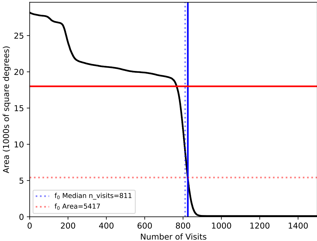
noroll_mjdp60_v3.4_10yrs : f0
