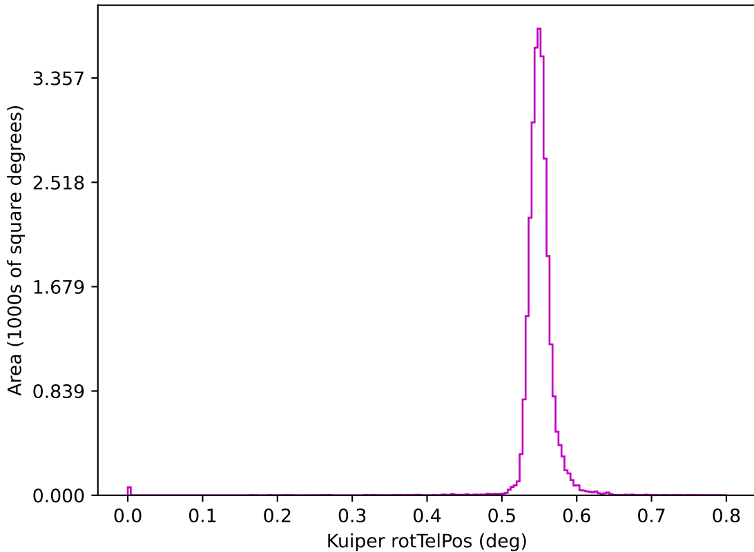
noroll_mjdp60_v3.4_10yrs z: Kuiper rotTelPos
