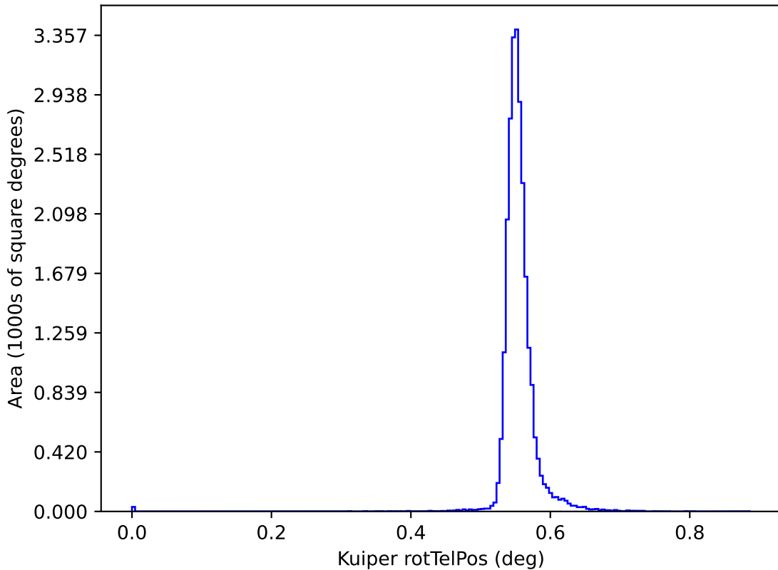
noroll_mjdp60_v3.4_10yrs y: Kuiper rotTelPos
