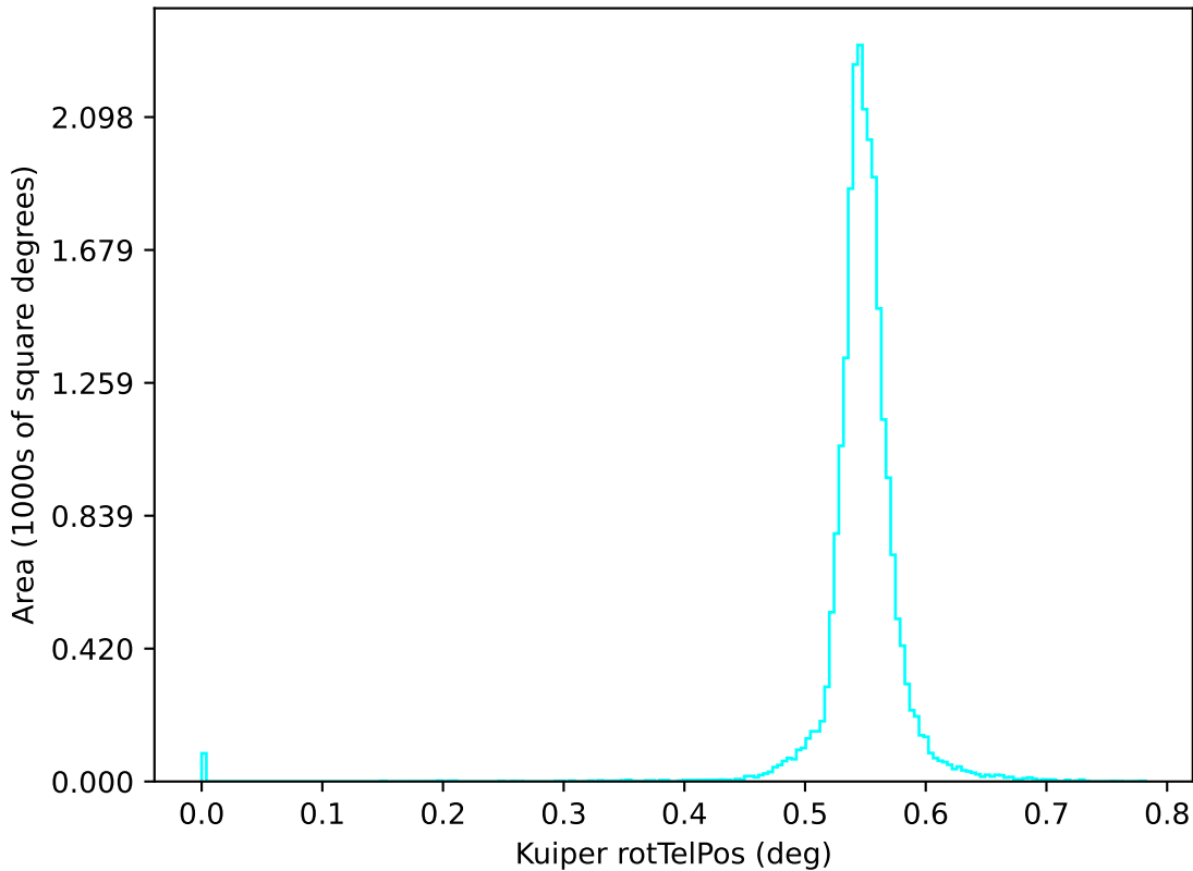
noroll_mjdp60_v3.4_10yrs u: Kuiper rotTelPos
