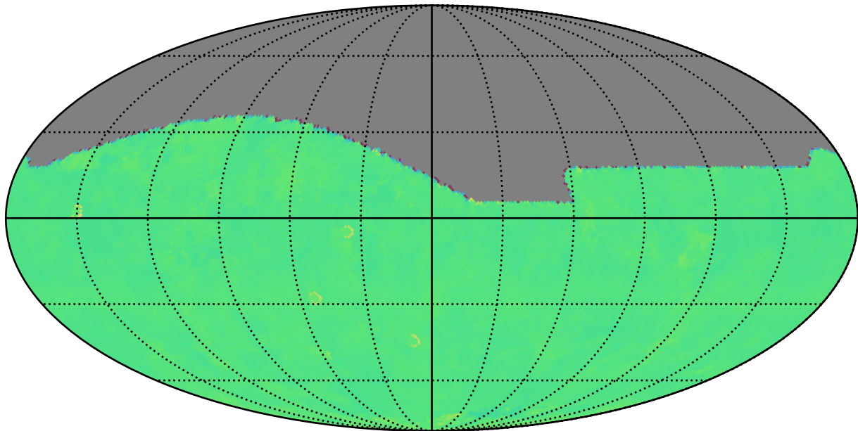
noroll_mjdp60_v3.4_10yrs i: Kuiper rotTelPos
