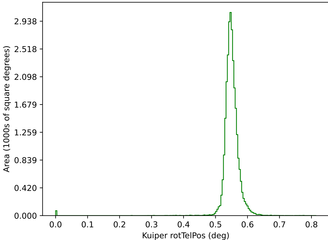
noroll_mjdp60_v3.4_10yrs g: Kuiper rotTelPos
