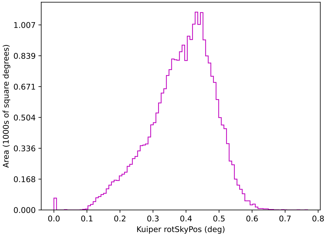
noroll_mjdp60_v3.4_10yrs z: Kuiper rotSkyPos
