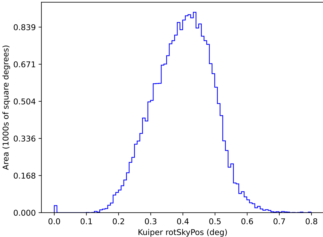
noroll_mjdp60_v3.4_10yrs y: Kuiper rotSkyPos
