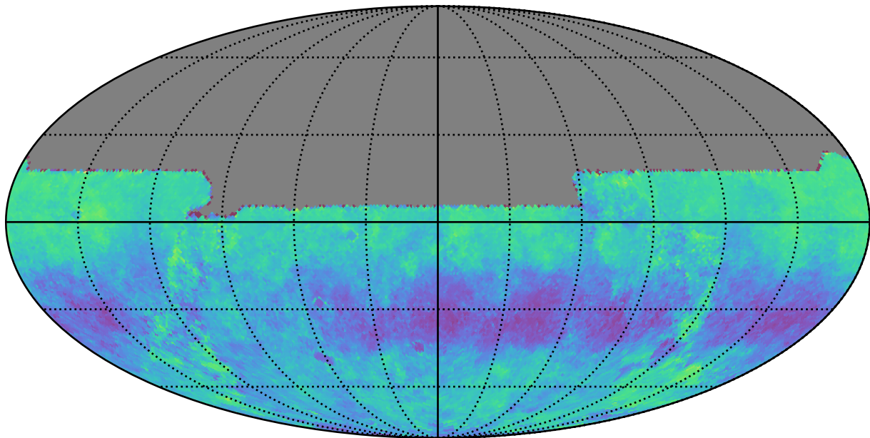
noroll_mjdp60_v3.4_10yrs u: Kuiper rotSkyPos
