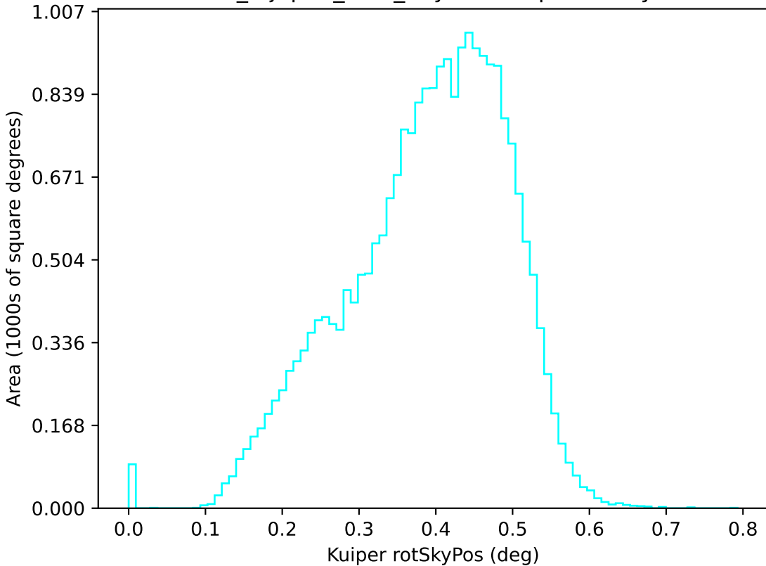
noroll_mjdp60_v3.4_10yrs u: Kuiper rotSkyPos
