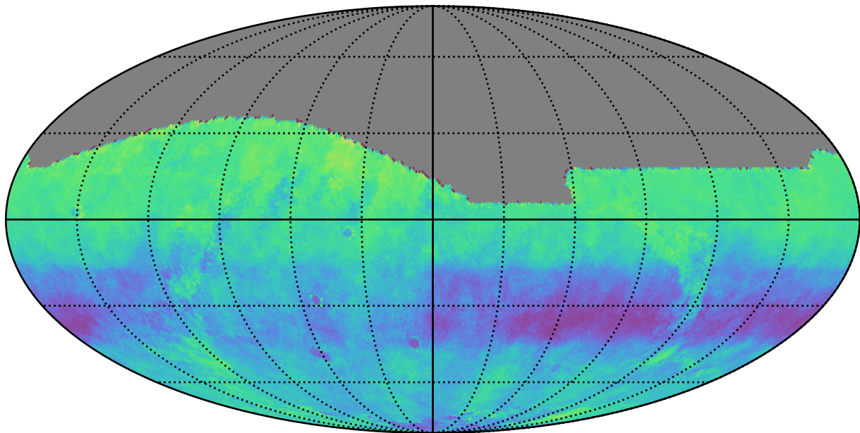
noroll_mjdp60_v3.4_10yrs r: Kuiper rotSkyPos
