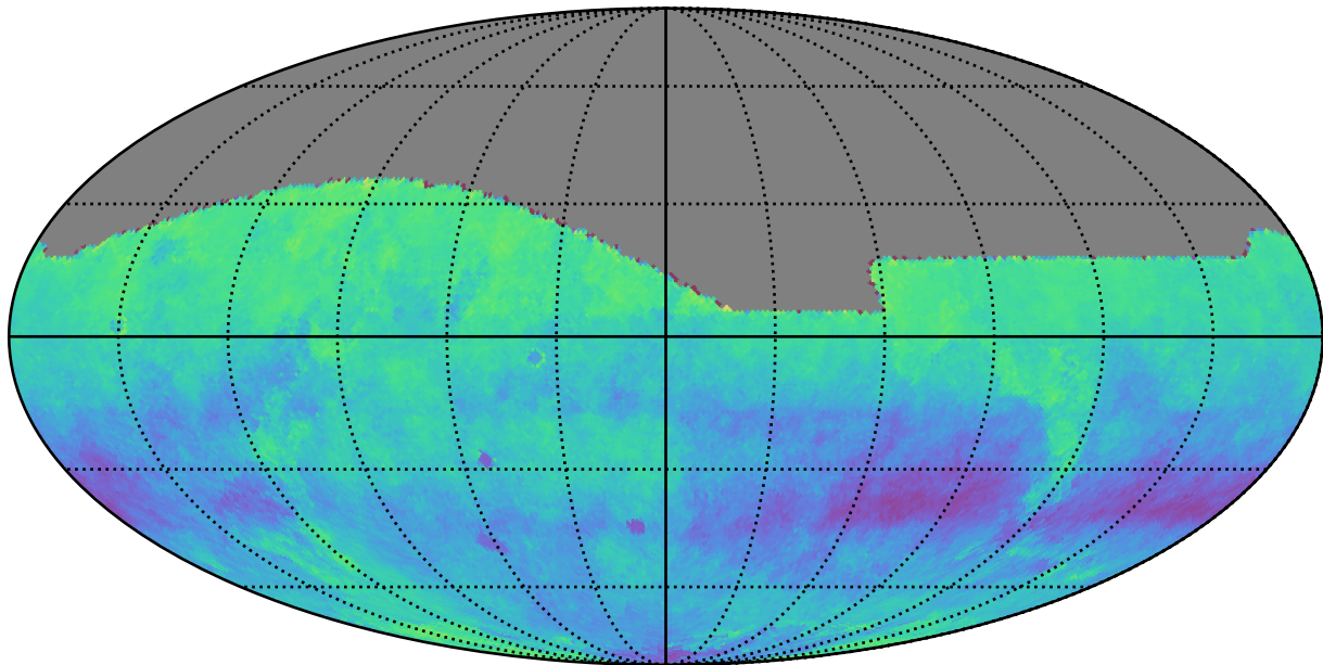
noroll_mjdp60_v3.4_10yrs i: Kuiper rotSkyPos
