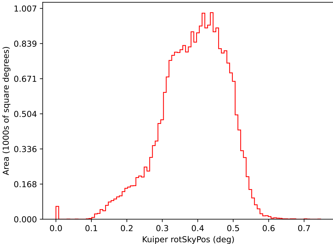
noroll_mjdp60_v3.4_10yrs i: Kuiper rotSkyPos
