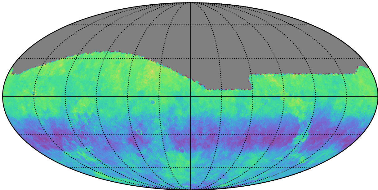
noroll_mjdp60_v3.4_10yrs g: Kuiper rotSkyPos
