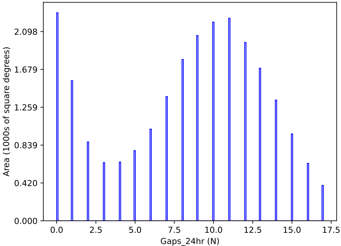
noroll_mjdp60_v3.4_10yrs y band: Gaps_24hr
