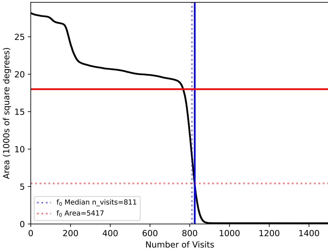
noroll_mjdp60_v3.4_10yrs All sky: f0
