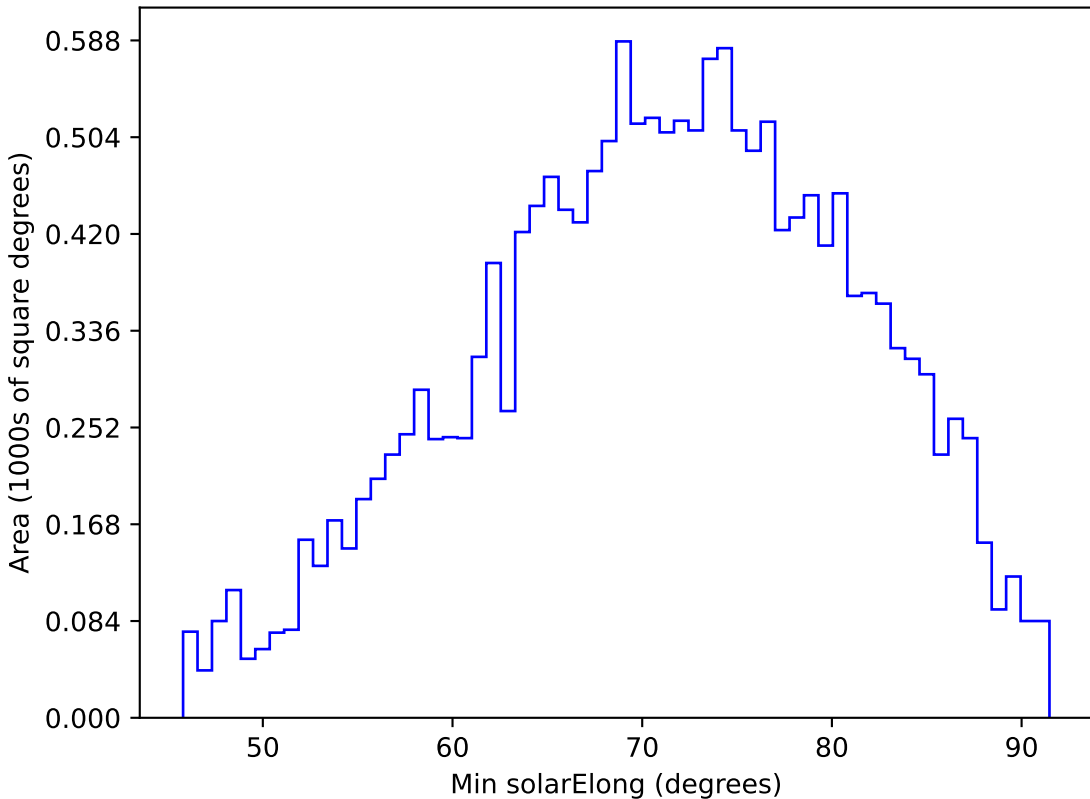
noroll_mjdp60_v3.4_10yrs WFD y band: Min solarElong
