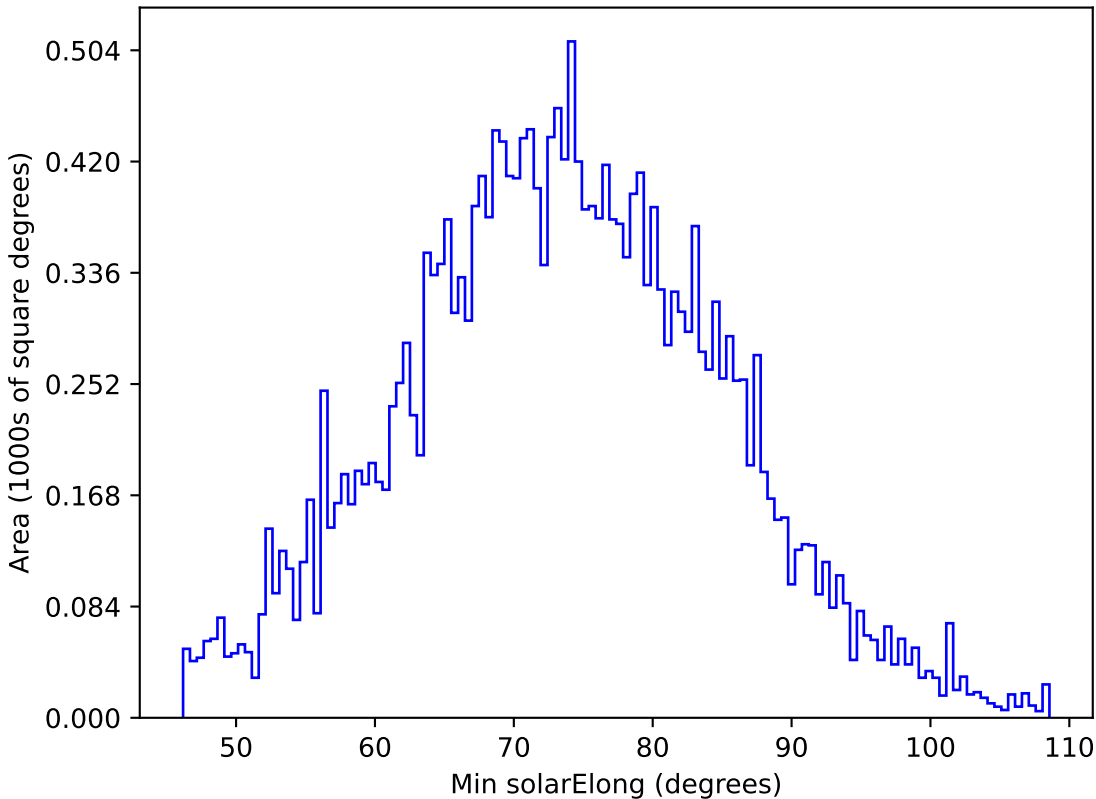
noroll_mjdp60_v3.4_10yrs All sky y band: Min solarElong
