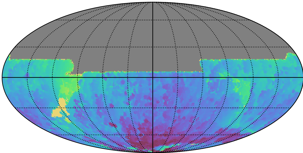
noroll_mjdp60_v3.4_10yrs All sky y band: Min HA
