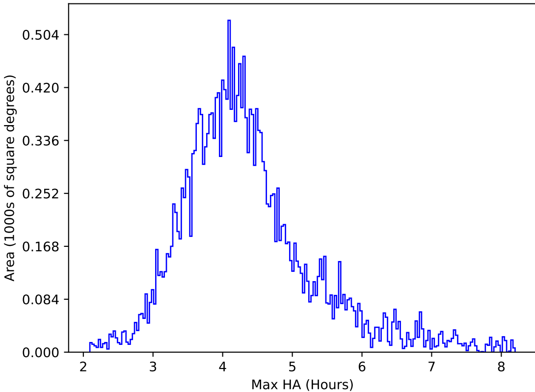
noroll_mjdp60_v3.4_10yrs All sky y band: Max HA
