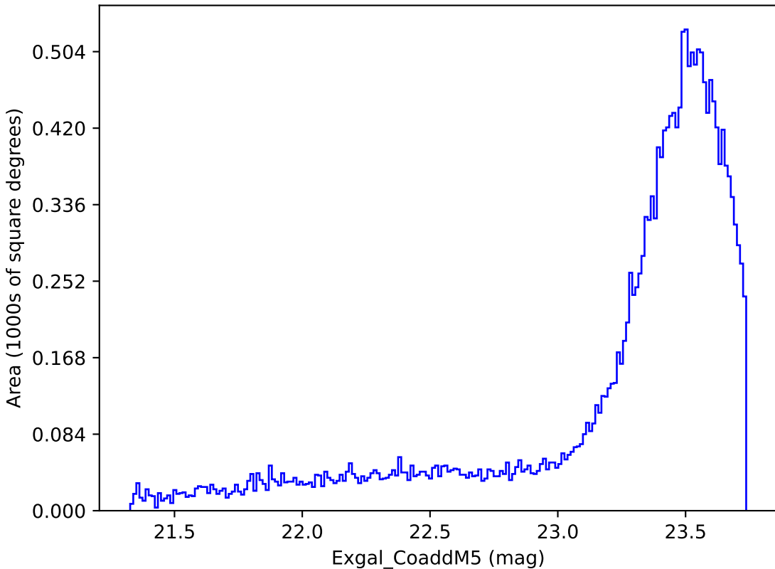
noroll_mjdp60_v3.4_10yrs Yr 3-4 y band: Exgal_CoaddM5
