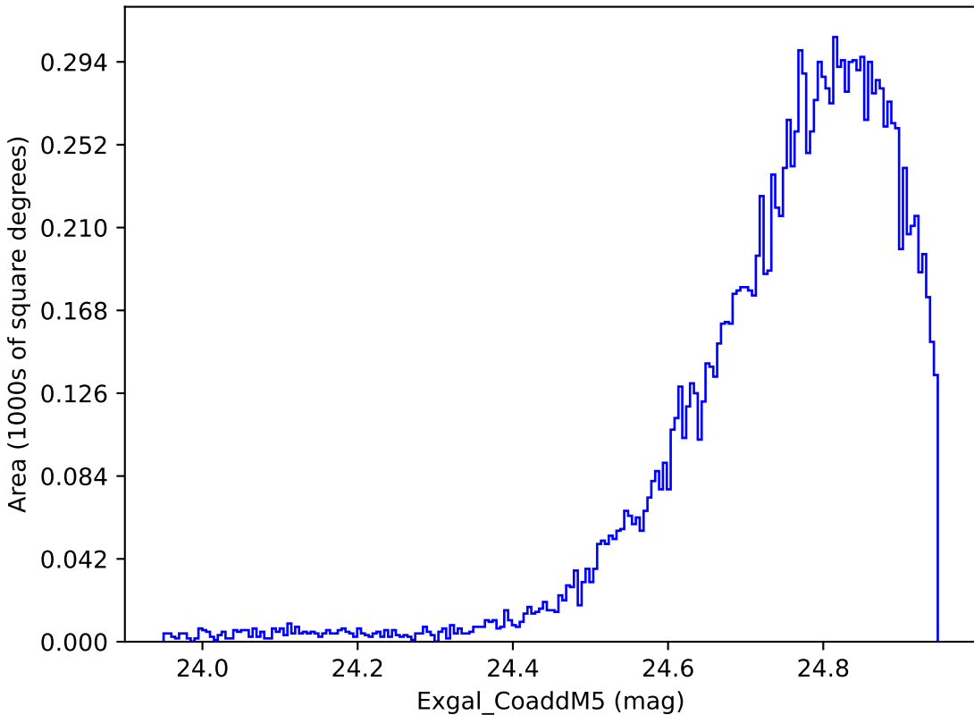
noroll_mjdp60_v3.4_10yrs WFD y band: Exgal_CoaddM5
